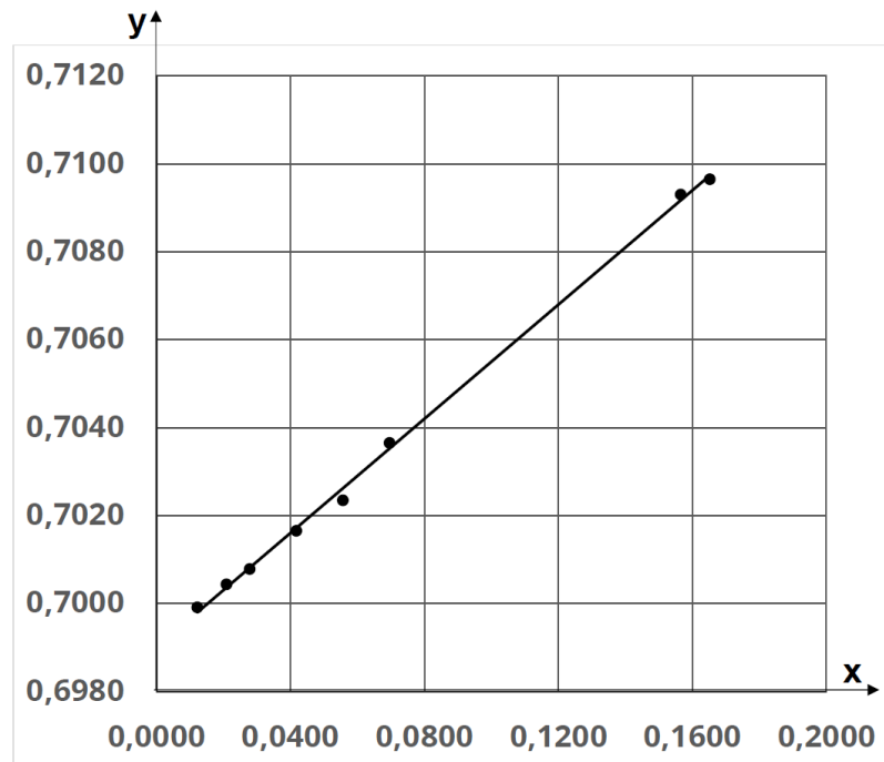
Figure 1 : Évolution du rapport y = \frac{N(^{87}_{38}\text{Sr})}{N(^{86}_{38}\text{Sr})} en fonction du rapport x = \frac{N(^{87}_{37}\text{Rb})}{N(^{86}_{38}\text{Sr})}
